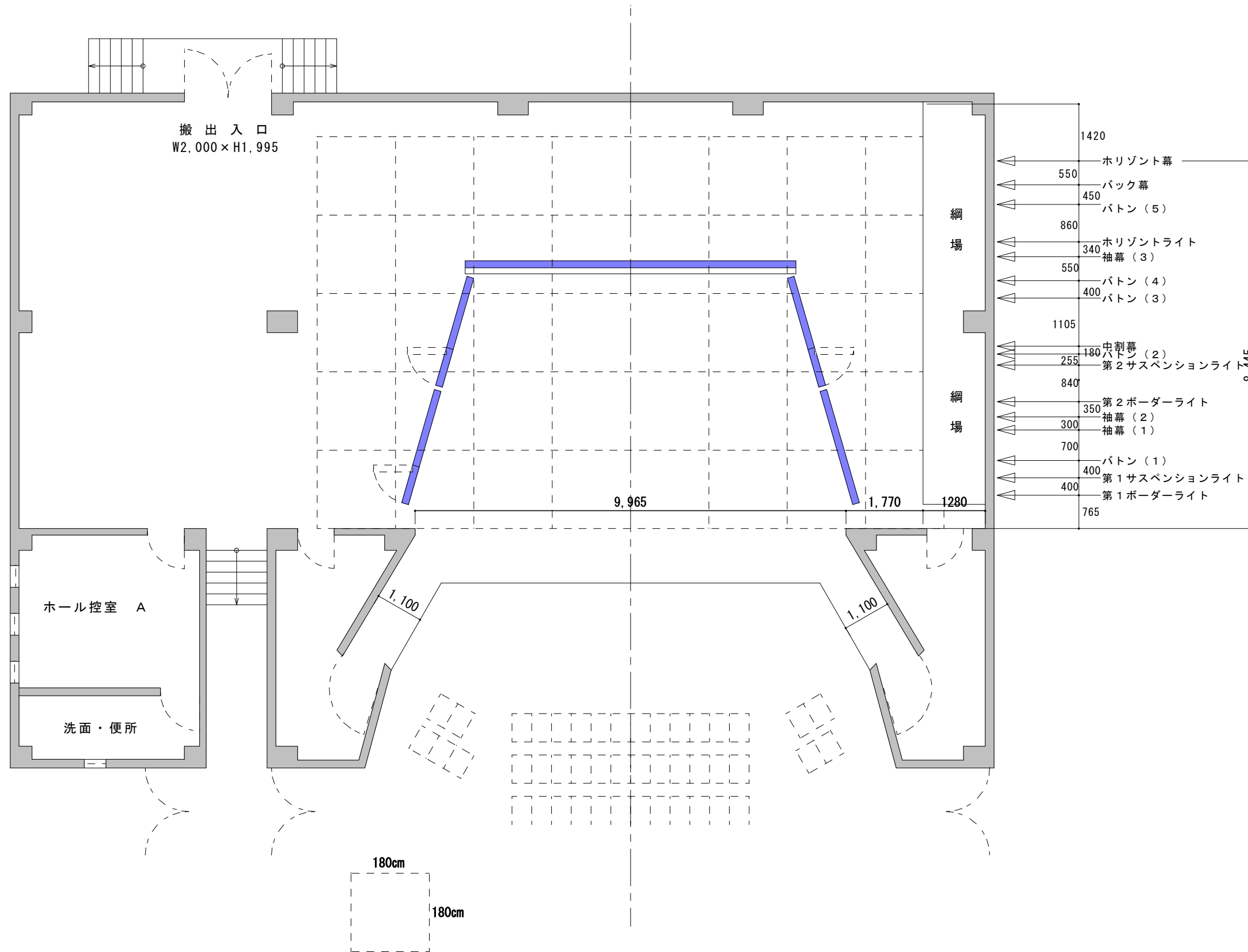
ビバホール 舞台平面図
