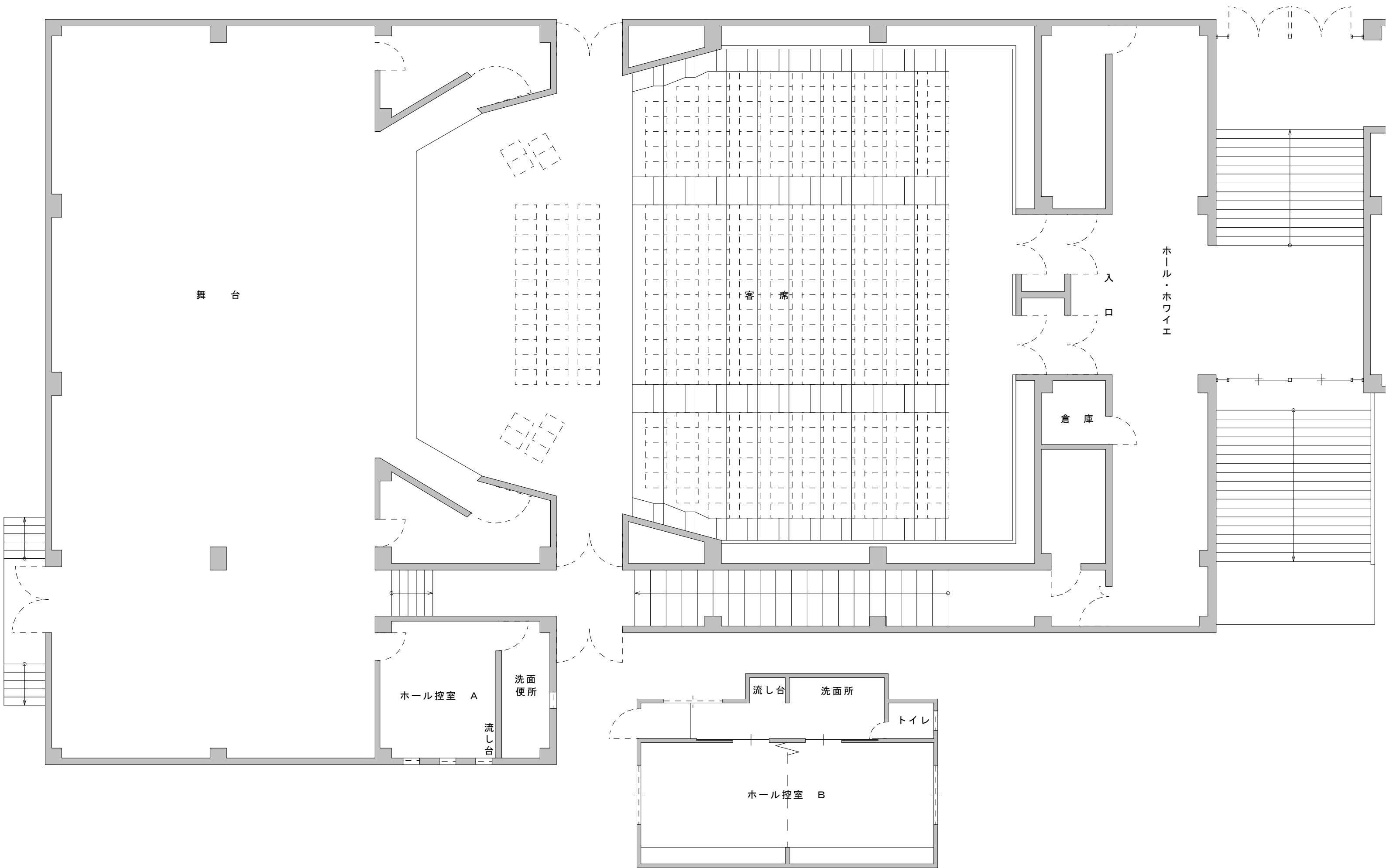
ビバホール 平面図
